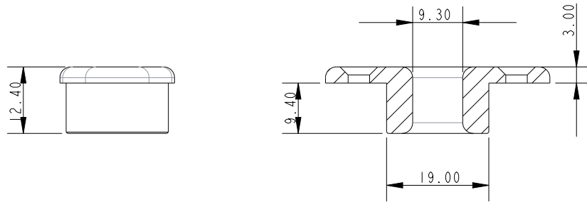
SECTION XSEC0001-XSEC0001
