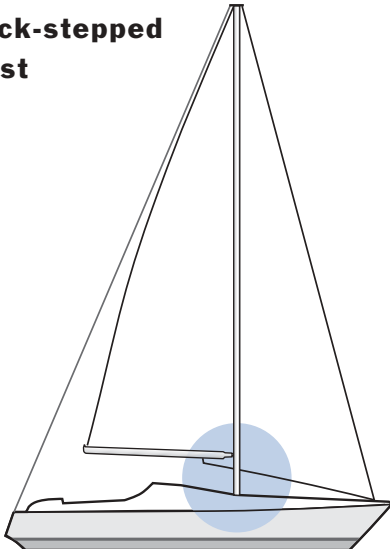
Keel-stepped mast
